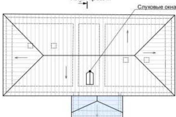
План кровли
